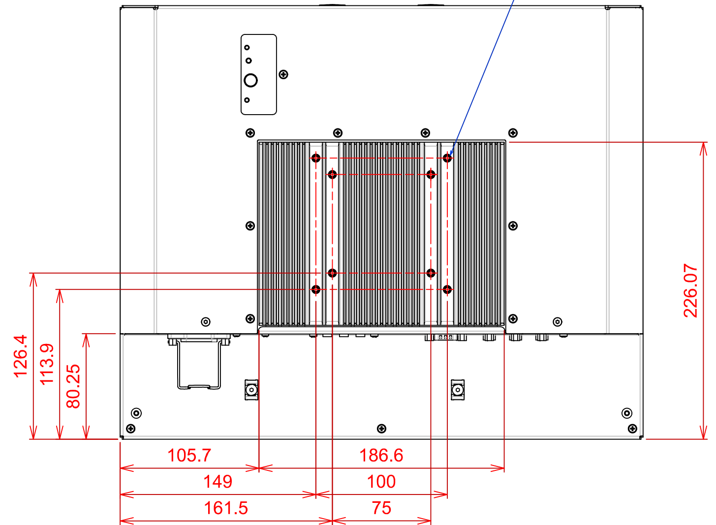
VUE ARRIERE
