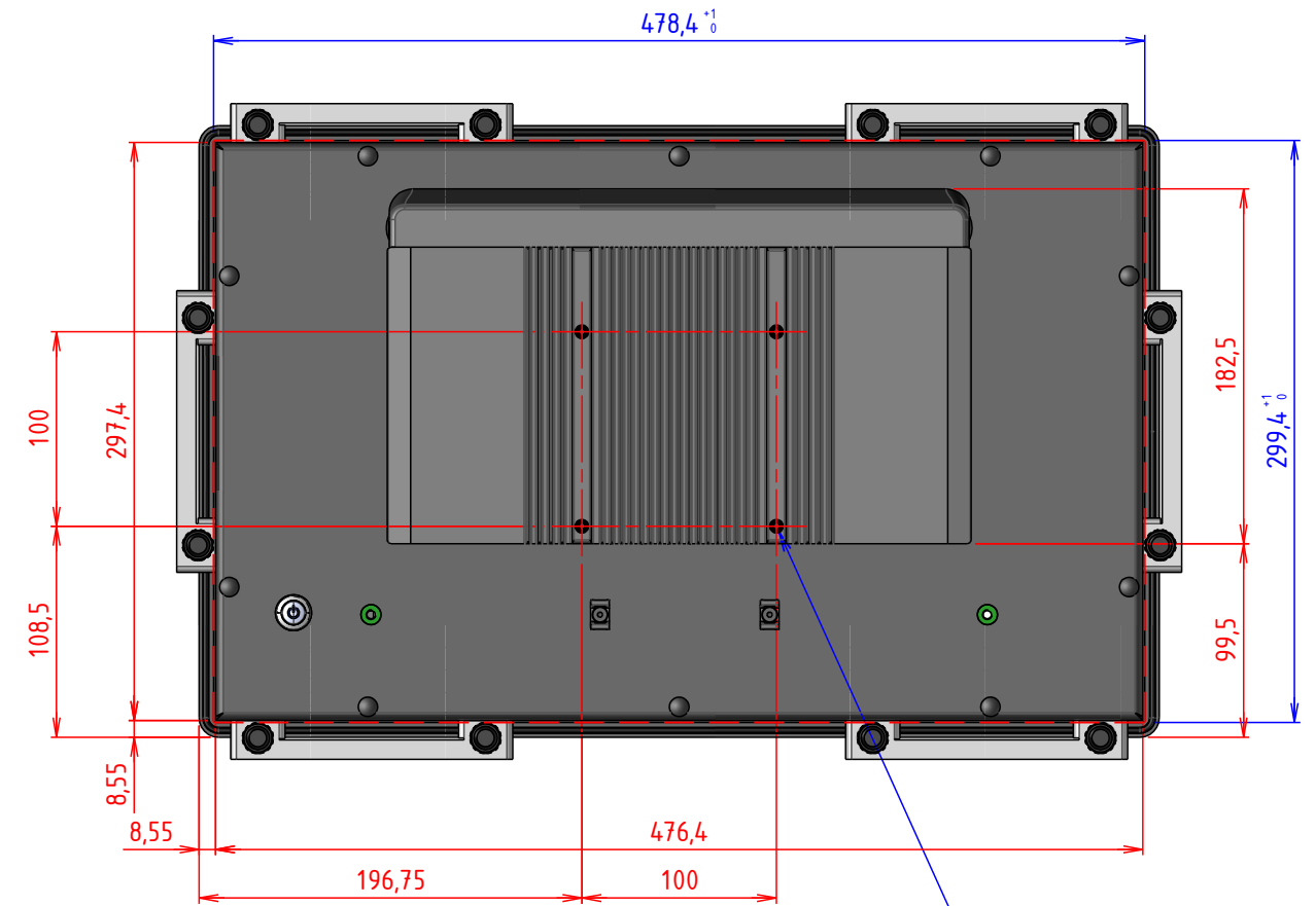
VUE ARRIERE
