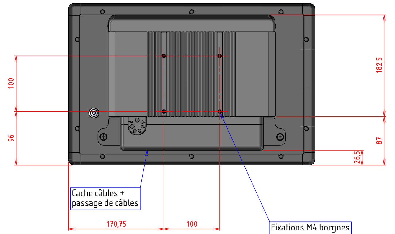
VUE ARRIERE
