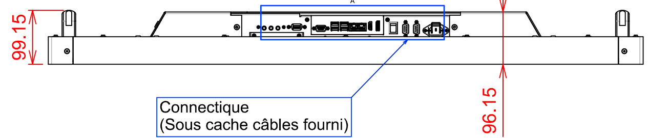
VUE DE DESSOUS A
